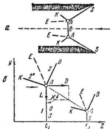
Рис. 2. Неправильные тройные ударные маховские конфигурации, возникающие: a – при сверхзвуковом обтекании двух параллельных плоских клиньев; б – при детонации; SA – падающая волна; AK – отраженная волна; AB – «третья волна», «маховская волна», «излом»
