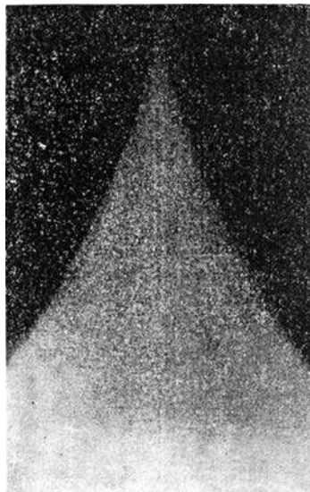
Рис. 1. Прямая фоторегистрация процесса распространения пламени в смеси 33,0\%C_2H_2 + 67,0\%O_2 (по объему)
