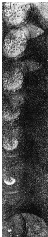
Рис. 2. Последовательные фотографии процесса распространения пламени в смеси ацетилена с кислородом ( 37,5\%C_2H_2 + 62,5\%O_2 )
