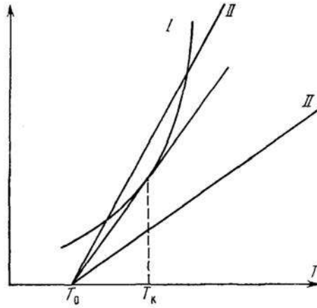
Рис. 1. К нестационарной теории теплового взрыва ( I – кривая теплоприхода вследствие химической реакции; II – кривая теплоотвода через стенки реакционного сосуда)
