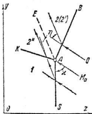
Рис. 3. Тройная ударная конфигурация и течение газа в окрестности тройной точки A в системе координат, связанных с этой точкой для пульсирующей детонации.
