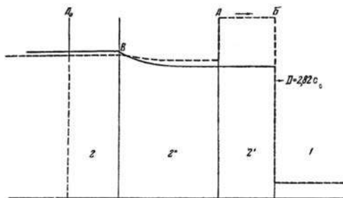
Рис. 2. Распад разрыва на ударную волну и волну разрежения:
