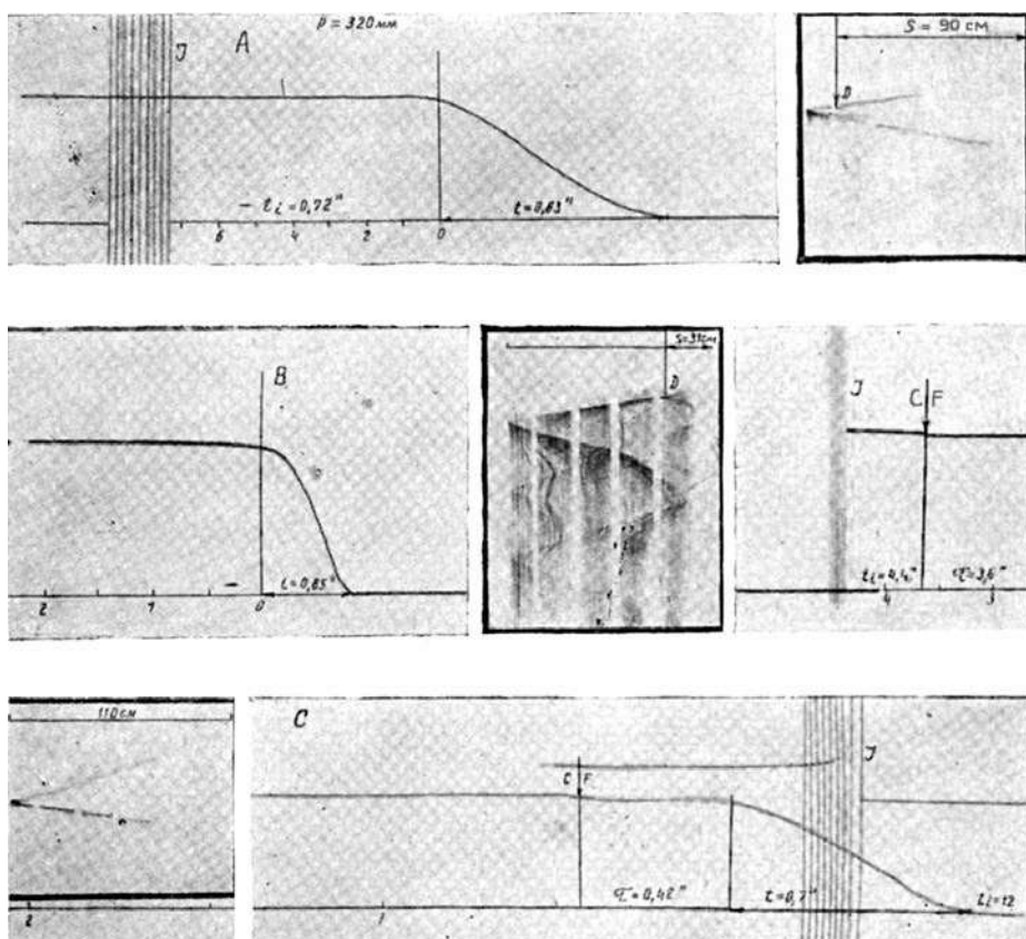
Рис. 2. 1 – момент искрового зажигания; CF – холодное пламя; D – начало детонации
