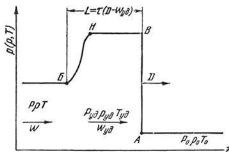
Рис. 3. Схема детонации как комплекса: ударная волна – зона реакции:
