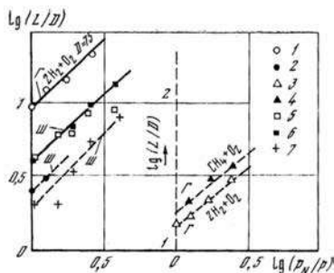
Рис. 5. Результаты опытов, изображенных на графиках рис. 1–4, в логарифмических координатах
