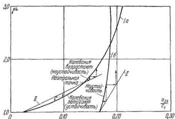
Рис. 26. К нелинейной теории пульсаций в камерах сгорания (I — зависимости перепада давления в ударной волне — волне давления — от скорости пламени; II — зависимости скорость пламени от перепада давления в ударной волне — волне давления)
