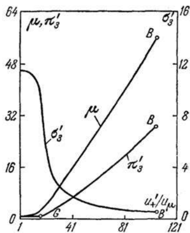
Рис. 24. Зависимость давления в ударной волне, давления и плотности продуктов сгорания при нестационарных режимах горения в открытой трубе от безразмерной скорости пламени по частицам стехиометрической метанокислородной смеси (обозначения те же, что и на рис. 22)
