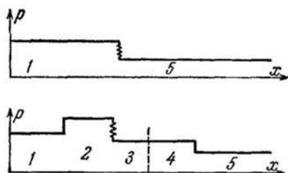
Рис. 25. Распад разрыва, возникшего от увеличения скорости пламени по частицам в слабой дефлаграции (1 – несгоревший газ; 5 – продукты сгорания стационарной слабой дефлаграции; 2 и 4 – газ в ударных волнах, возникших при увеличении скорости пламени; 3 – продукты сгорания за фронтом дефлаграции после распада разрыва)
