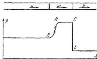
Рис. 9. Схематическое распределение давления в детонации, рассматриваемой как комплекс из ударной волны и зоны воспламенения
