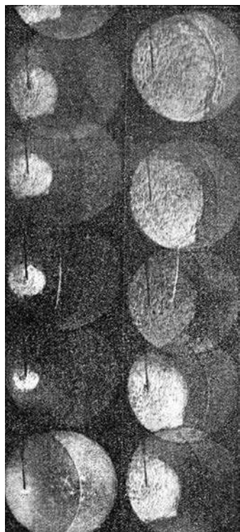
Рис. 4. Последовательные фотографии процесса распространения пламени в смеси ацетилена с кислородом (37,5%С 2 Н 2 + 62,5%О 2 )
