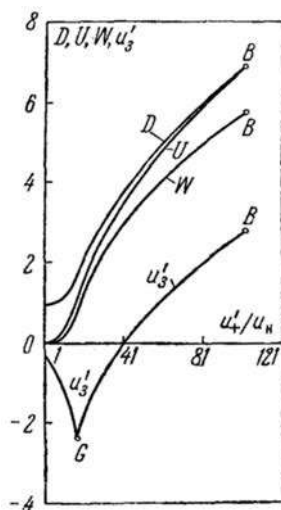
Рис. 23. Зависимость величин, характеризующих режимы нестационарного горения при зажигании у открытого конца трубы, от безразмерной скорости пламени по частицам стехиометрической метанокислородной смеси ( \gamma Q/c_0^2 = 44,5 ; \gamma = 1,31 ; обозначения те же, что и на рис. 21)
