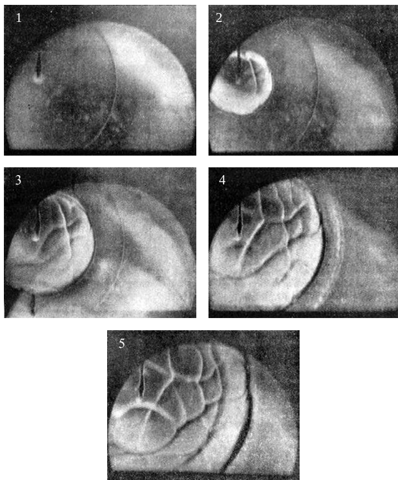
Рис. 9. Последовательные фотографии процесса распространения пламени в медленно горящей смеси 10% саратовского газа и 90% воздуха
