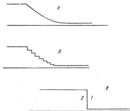
Рис. 1. Образование разрыва состояния и скорости газа:
