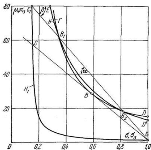
Рис. 6. Кривые Гюгонио ( H – для исходного состояния C_1 , G – для исходного состояния A ; кривые H и G всегда пересекаются в точках, лежащих на прямой, соединяющей исходные состояния C_1 и A )
