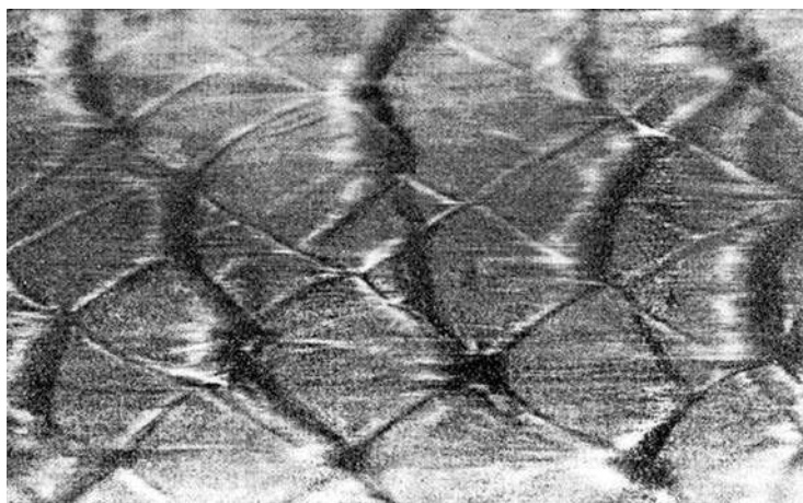
Рис. 8. След «нормальной» детонации на закопченной поверхности трубы. Волна распространяется справа налево
