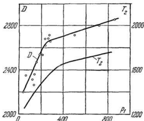
Рис. 13. Зависимость скорости детонации D (м/сек) и температуры T_2 (°K) за ударным фронтом от начального давления p_1 (мм рт. ст.) смеси 2\text{H}_2 + \text{O}_2 (диаметр трубы 16 мм)
