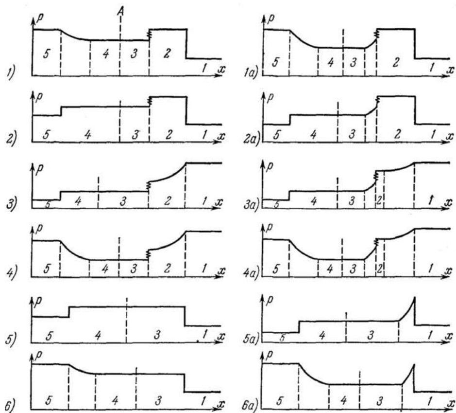
Рис. 19. Все возможные случаи распада произвольного теплового разрыва по Г.М. Бам-Зеликовичу (слева без волны разрежения за фронтом горения – слабая дефлаграция и сильная детонация; справа с волной разрежения – дефлаграция и детонация Чепмена – Жуге; случаи 1 – 4 относятся к дефлаграции, 5 и 6 – к детонации)
