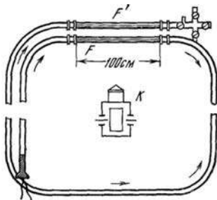
Рис. 1. Схема установки
