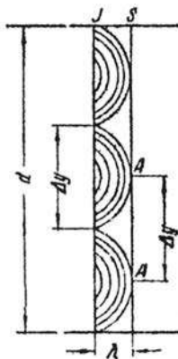
Рис. 6. Схема распространения возмущений от фронта воспламенения J и появления изломов в переднем ударном фронте S (к выводу зависимости среднего размера неоднородности во фронте детонаций от газодинамических и кинетических факторов)
