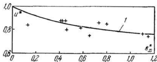
Рис. 15. Зависимость безразмерной скорости детонации u^* = u_{0*} \sqrt{2(\gamma^2 - 1)q} в шероховатой трубе от коэффициента сопротивления c_x^0 = c_x \sqrt{2(\gamma^2 - 1)q} / u_p (1 – теоретический расчет; экспериментальные точки построены на основании опытов К.И. Щелкина для смесей водорода и этана с кислородом).
