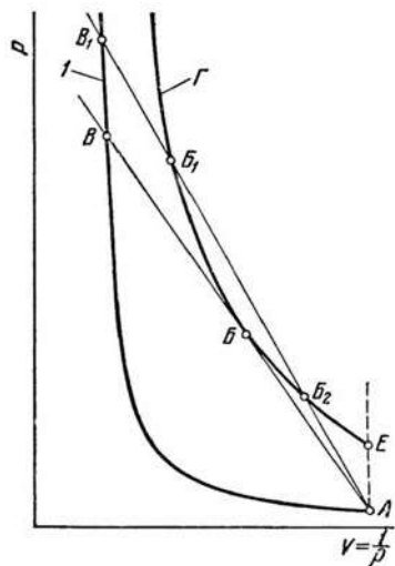
Рис. 2. p , V – диаграммы: I – для ударной волны; \Gamma – для продуктов детонации; A – исходная точка для обеих кривых
