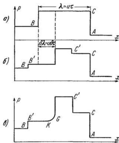
Рис. 10. Возникновение двух ударных волн C' и B' при сокращении периода задержки воспламенения во фронте детонации на \delta\tau .
