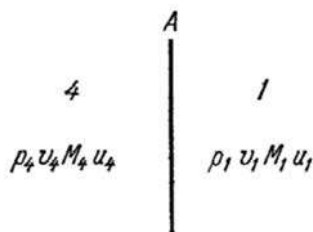
Рис. 17. К теории распада произвольного разрыва (плоскость разделяет газы I и 4 , обладающие различными давлением p , удельным объемом v , молекулярным весом M и скоростью движения)
