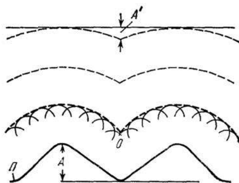
Рис. 3. Уменьшение амплитуды начального искривления пламени от A до A' благодаря выравнивающему действию распространения пламени (эффект Гюйгенса)
