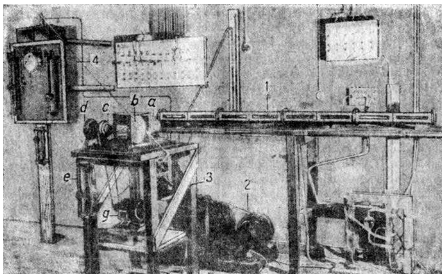
Рис 3. Общий вид установки для фотографирования: 1 – труба; 2 – насос; 4 – искровая установка; 5 – фотоаппарат; а – объектив; б – барабан; с – передача; d – тахометр; е – реостат; g – мотор
