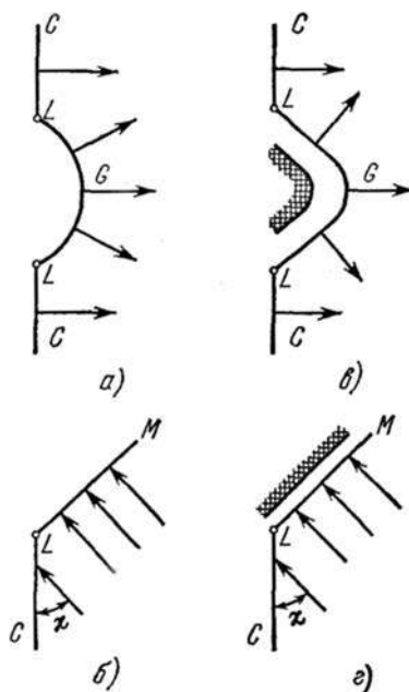
Рис. 12. Схема изломов ударного фронта детонации ( a , b – без горения непосредственно за изломом; v , z – с горением)
