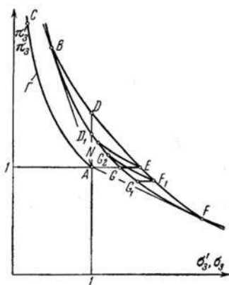
Рис. 20. Схематическое изображение адиабаты Гюгонио и кривых, построенных по обобщенной адиабате Гюгонио (кривая FG_1GG_2ND_1B – Q -кривая)
