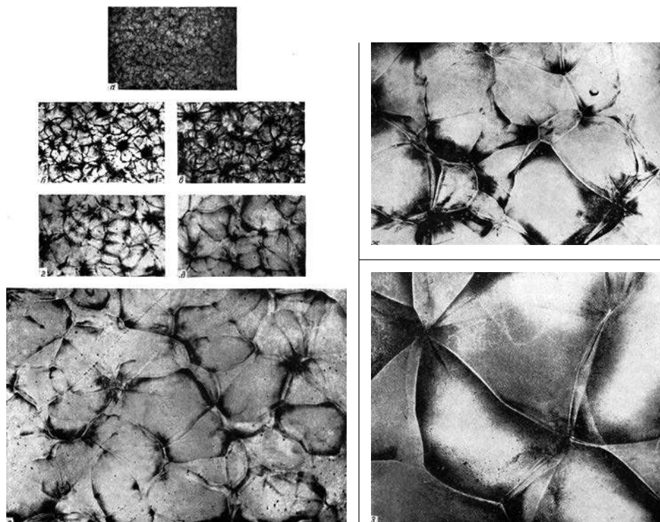
Рис. 8. Фотографии с отпечатков на закопченных стеклянных пластинках, оставленных волной детонации при различных начальных давлениях исходной смеси 2\text{H}_2 + \text{O}_2 : a - p_0 = 3 \text{ кг/см}^2 ; б - p_0 = 1 \text{ кг/см}^2 ; в - p_0 = 1 \text{ кг/см}^2 (сферическая детонация в резиновом шаре); г - p_0 = 500 \text{ мм рт. ст.} ; д - p_0 = 400 \text{ мм рт. ст.} ; е - p_0 = 300 \text{ мм рт. ст.} ; ж - p_0 = 200 \text{ мм рт. ст.} ; з - p_0 = 90 \text{ мм рт. ст.}
