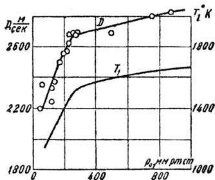
Рис. 10. Зависимость скорости детонации D и средней температуры T_1 за передним ударным фронтом волны от начального давления смеси 2\text{H}_2 + \text{O}_2 (диаметр трубы 16 мм)
