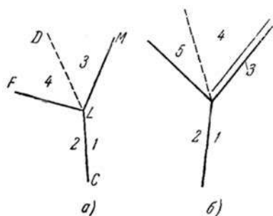
Рис. 11. Тройная маховская конфигурация (излом) в случае пересечения двух ударных волн CL и LM (а) и пересечения ударной волны с детонацией (б)
