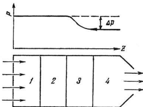
Рис. 9. Упрощенная схема ракетной камеры сгорания: 1–2 – зоны смешения топлива с окислителем и подогрева смеси; 3 – зона реакции; 4 – продукты сгорания
