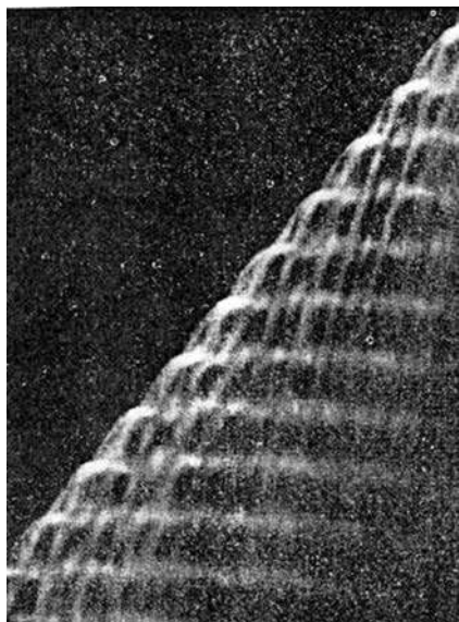
Рис. 4. Фотография спиновой детонации на движущуюся пленку. Волна распространяется справа налево
