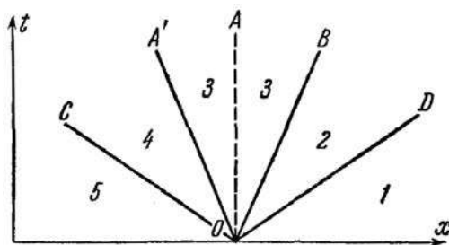
Рис. 18. Изображение распада произвольного теплового разрыва в плоскости x - t (OA – начальное положение разрыва; OD – ударная волна – волна разрежения; OB – дефлаграция; OA' – движение контактного разрыва; OC – ударная волна – волна разрежения)
