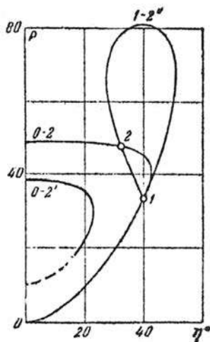
Рис. 5. Результаты численного расчета тройной конфигурации для пульсирующей детонации, показывающие что детонационная поляра 0–2' и ударная поляра 1–2'' не пересекаются
