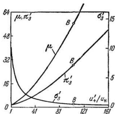
Рис. 22. Зависимость давления в ударной волне \mu , давления \pi_3' и плотности \sigma_3' продуктов реакции от безразмерной скорости пламени в критическом режиме (дефлаграция Чепмена – Жуге) в стехиометрической метано-кислородной смеси
