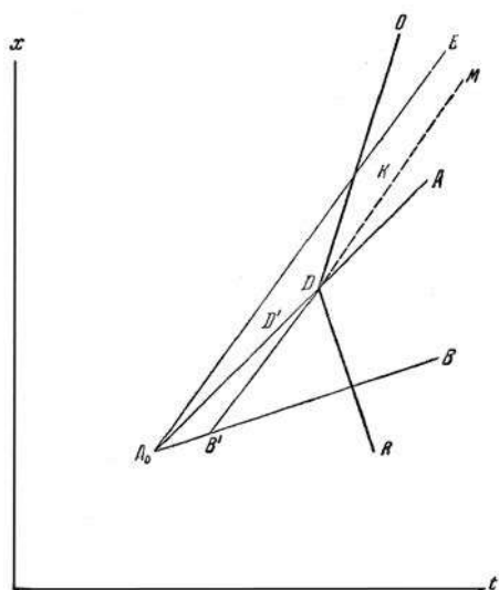
Рис. 4. Образование второй ударной волны и возникновение детонации непосредственно вблизи фронта пламени
