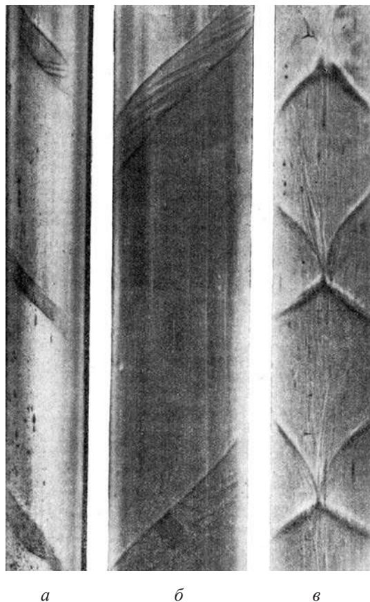
Рис. 7. Следовые отпечатки детонации смеси 2\text{H}_2 + \text{O}_2 : а , б – спиновой; p_0 = 50 мм рт. ст.; d = 16 мм; G для а = 1,3; б = 2,25; в – пульсирующей с n = 2 ; p_0 = 130 мм рт. ст.; d = 11 мм; G = 2,5
