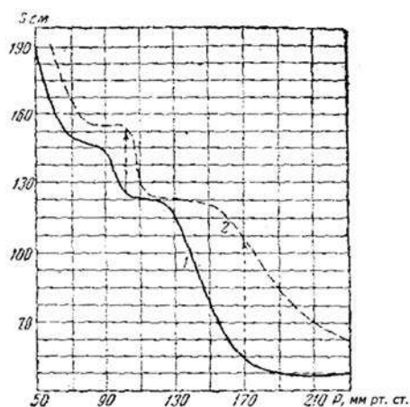
Рис. 3. 1 – C_5H_{12} + 8O_2 + 2N_2 ; 2 – C_5H_{12} + 8O_2 + 2N_2 + 1,2\% \text{ ТЭС}
