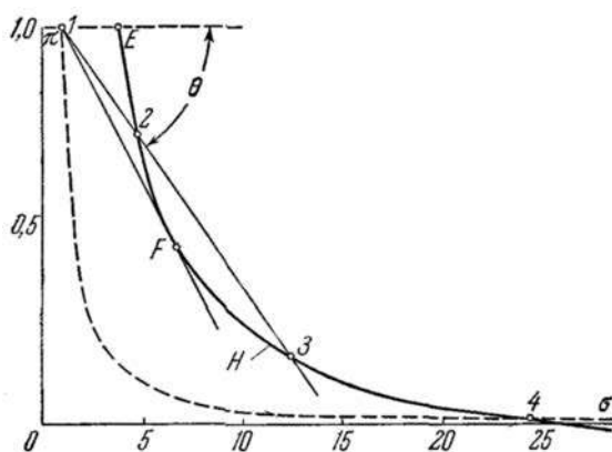
Рис. 7. Дефлаграционная часть кривой Гюгонио
