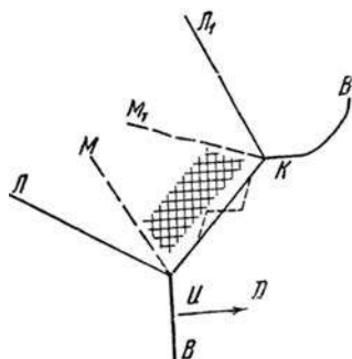
Рис. 7. Симметричный косой детонационный скачок: KL_1 – ударная волна, KM_1 – тангенциальный разрыв; остальные обозначения – те же, что и на рис. 6
