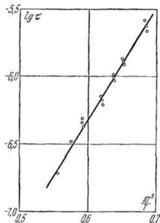
Рис. 14. Температурная зависимость запаздывания воспламенения бензола-кислородной смеси в детонационной волне \lg \tau сек – 10^3/T °K (видимая энергия активации в этих условиях равна 37 ккал/моль)
