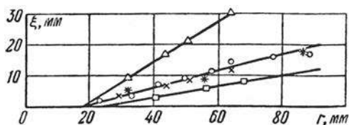
Рис. 7. Высота выпуклостей во фронте пламени \xi в мм в зависимости от радиуса пламенной сферы r в мм
