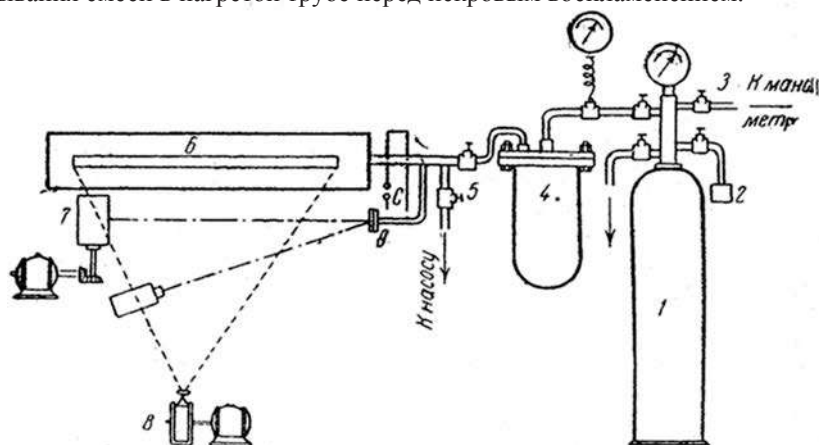
Рис. 1. Схема установки
