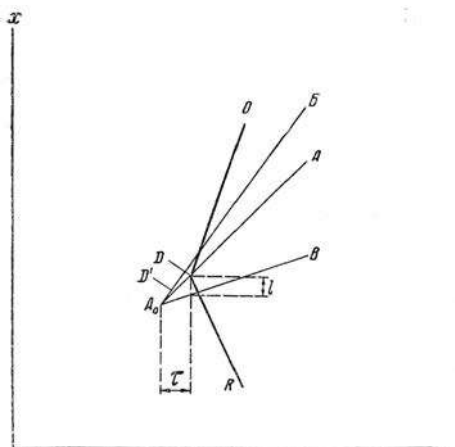
Рис. 3. Возникновение детонации впереди фронта пламени
