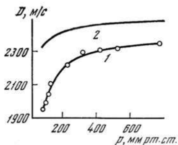
Рис. 3. Изменение скорости детонации с давлением для смеси \text{CH}_4 + 2\text{O}_2 : 1 — экспериментальная; 2 — вычисленная кривая; точки — данные Диксона
