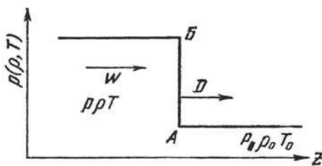
Рис. 1. Схема детонационной волны: p_0 , \rho_0 , T_0 – давление, плотность и температура исходного газа; p , \rho , T – продуктов сгорания; D – скорость фронта детонации; AB – скорость продуктов горения
