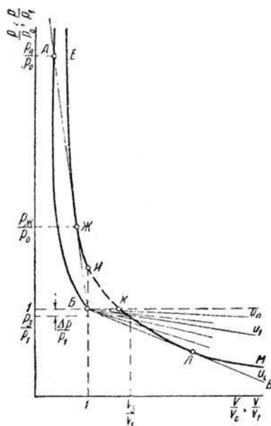
Рис. 2. Адиабаты Гюгонио
