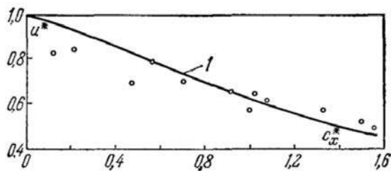
Рис. 16. Зависимость безразмерной скорости детонации u^* в шероховатой трубе от коэффициента сопротивления c_x^* (1 – теоретический расчет; экспериментальные точки построены по данным опытов П. Лаффита для смесей ацетилена и пропана с кислородом).
