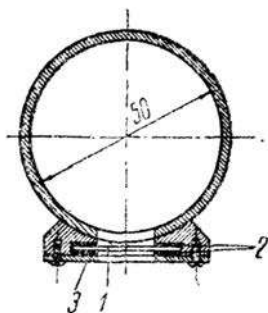
Рис. 1. Сечение трубы: 1 – окно; 2 – резиновые уплотнения; 3 – прижимная рамка
