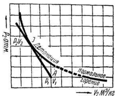
Рис. 4. Кривая Hugoniot
