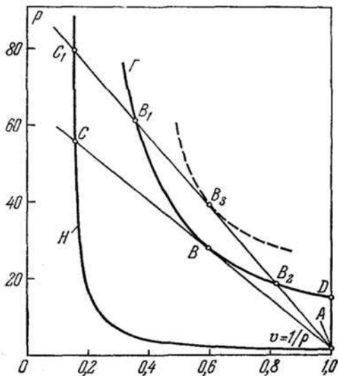
Рис. 5. Детонационная ветвь кривой Гюгонио
