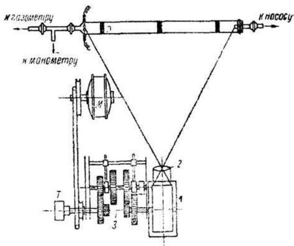
Рис. 2. Схема аппарата для фотографирования: 1 — барабан; 2 — объектив; 3 — передача; Т — тахометр
