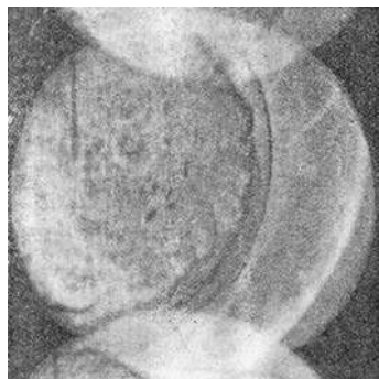
Рис. 3. Структура шарового пламени в смеси 50%С 2 Н 2 + 50%О 2 (1/2 натуральной величины)
