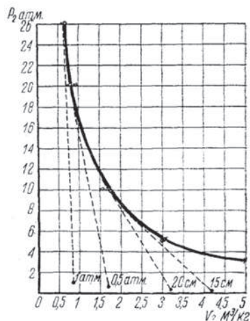
Рис. 6. Кривая Hugoniot для смеси \text{CH}_4 + 2\text{O}_2
