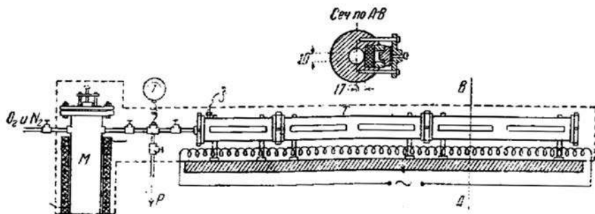
Рис. 1. Схема установки: М – смесительный баллон; Т – взрывная труба; с – свеча; р – к насосу
