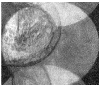
Рис. 5. Структура шарового пламени в смеси 37,5%С 2 Н 2 + 62,5%О 2 (кадр 6 из рис. 2; 1/2 натуральной величины)
