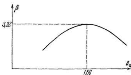
Рис. 2. К стационарной теории теплового взрыва (для сферического сосуда параметр \beta достигает максимума при \theta_{\text{ц}} = 1,60 ).
