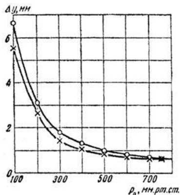
Рис. 9. Зависимость среднего размера неоднородности во фронте детонации от начального давления смеси 2\text{H}_2 + \text{O}_2 : верхняя кривая для трубы диаметром 30 мм; нижняя кривая для трубы диаметром 70 мм
