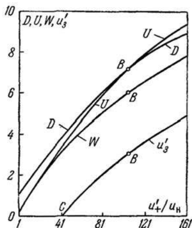
Рис. 21. Зависимость величин, характеризующих режимы нестационарного критического горения (дефлаграции Чепмена – Жуге) при зажигании у закрытого конца трубы, от безразмерной скорости пламени по частицам стехиометрической метано-кислородной смеси ( \gamma Q/c_0^2 = 44,5 ; \gamma = 1,31 ; D – скорость фронта ударной волны, предшествующей зоне горения; U – скорость фронта пламени относительно стенки трубы; W – скорость ударно-сжатого газа; u_3' – непосредственно за фронтом пламени)
