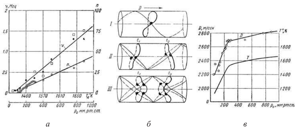
Рис. 8. Зависимости параметров детонационной волны от начального давления реагирующей смеси (смесь 2H_2 + O_2 , d = 16 мм):
