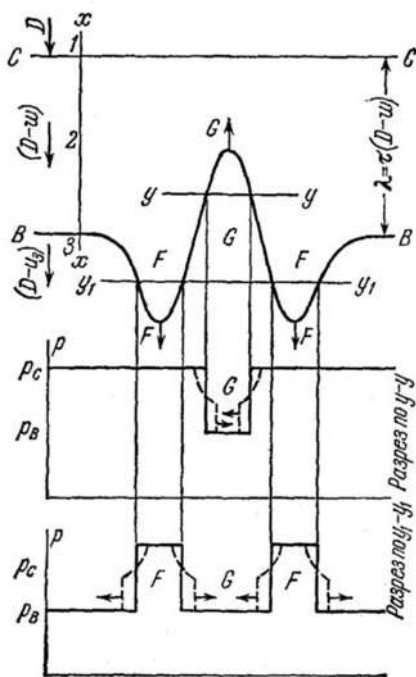
Рис. 8. Схема малого возмущения зоны воспламенения в детонации FGF (на рисунке сильно преувеличено; снизу, на разрезах, виден распад возмущения в направлении, поперечном к движению детонации)
